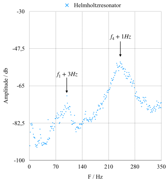
Abbildung 17: Fourier-Analyse im Bereich 0 \text{ Hz} bis 350 \text{ Hz}
